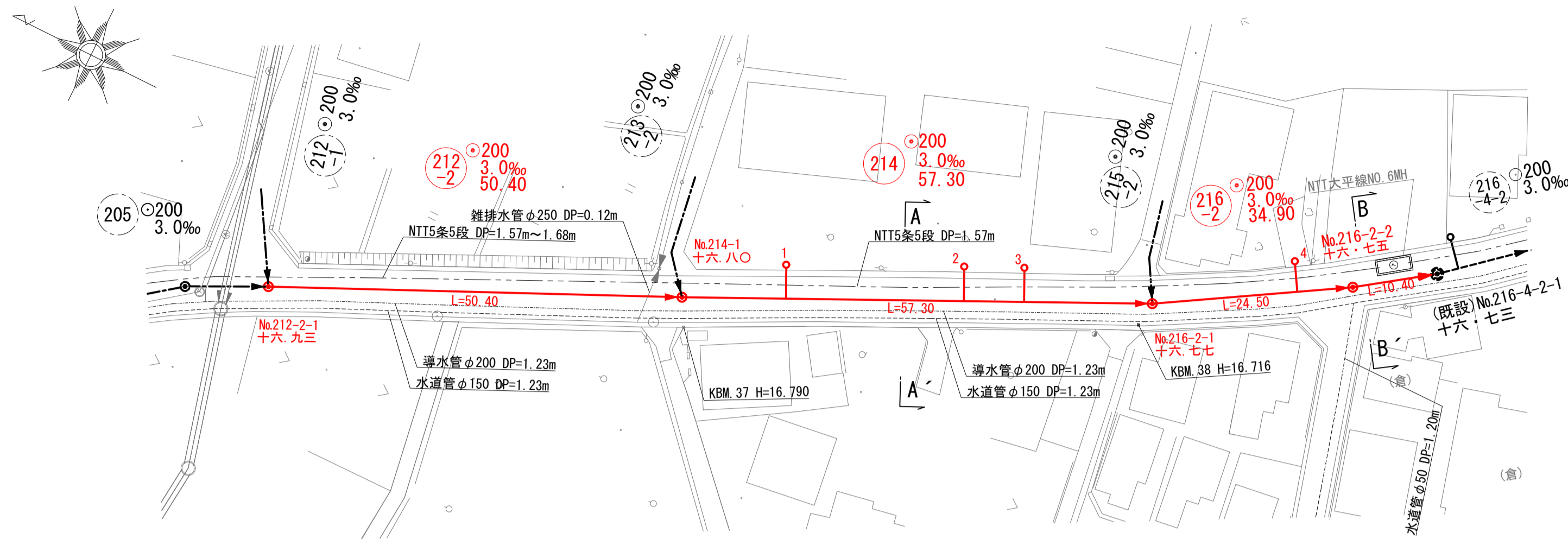
平面図 縮尺 1:500
