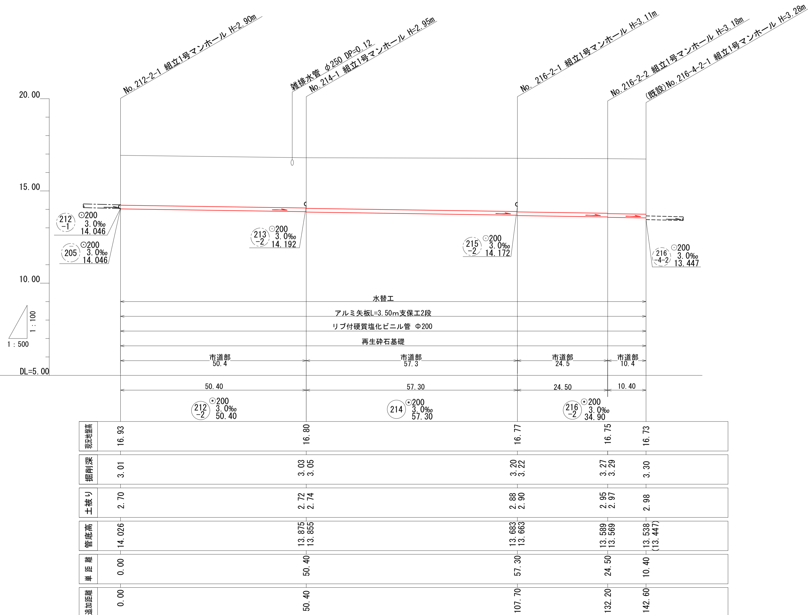
縦断面図 縮尺 縦 1:100 横 1:500
