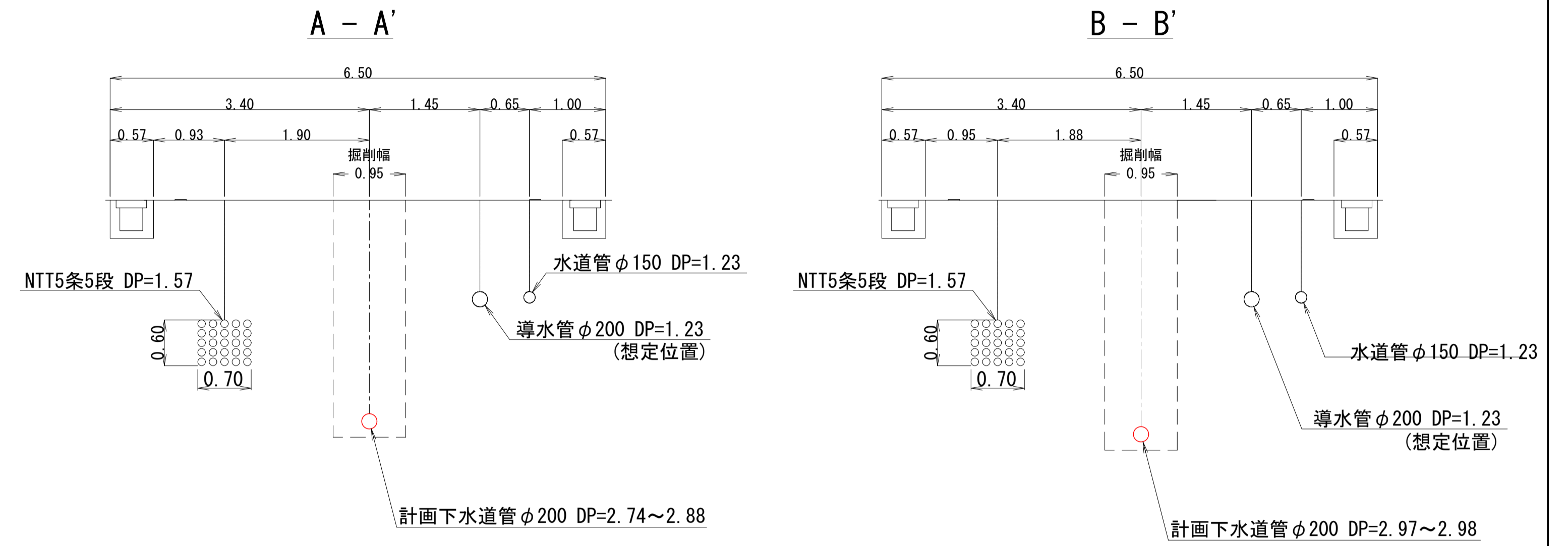
横断面図 縮尺 1:50
